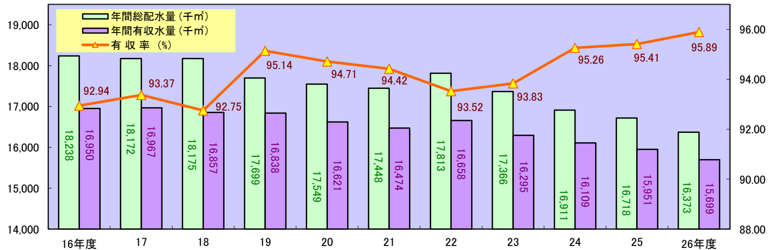
年間総配水量・年間有収水量・有収率の推移
