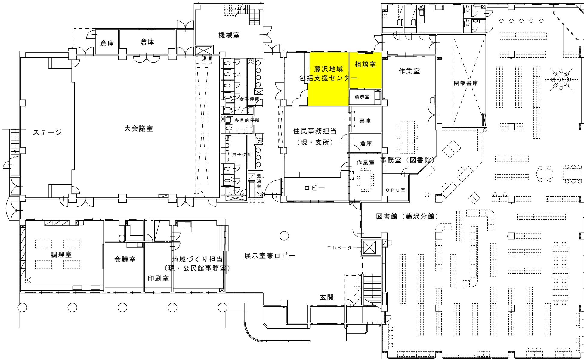
藤沢地区センター（現・藤沢支所・藤沢公民館） 1階平面図
