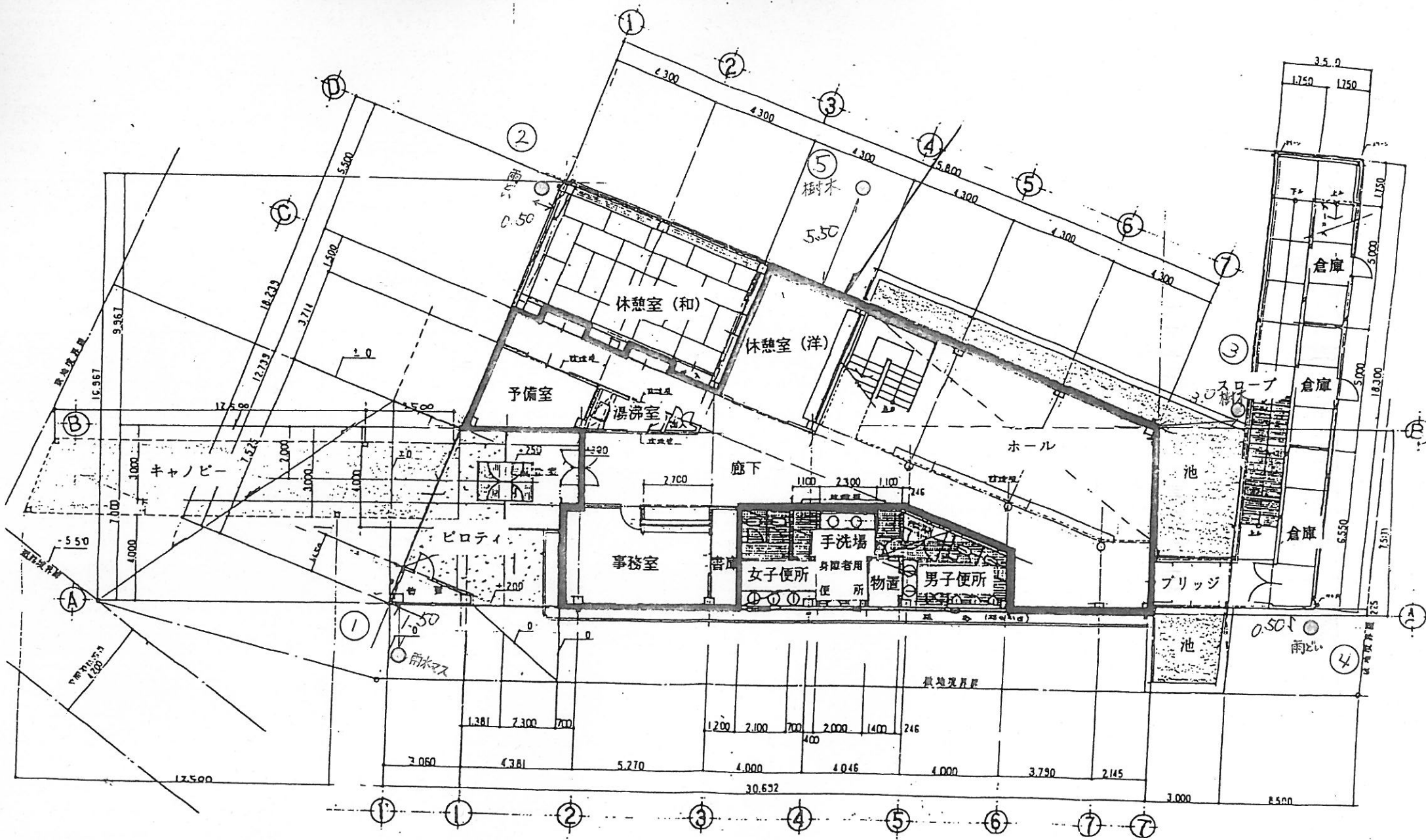
1階 平面図
