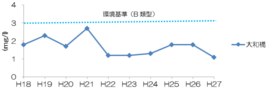
BOD (75%値)
