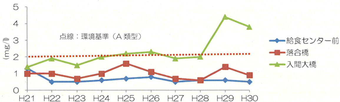
BOD（75%値）
