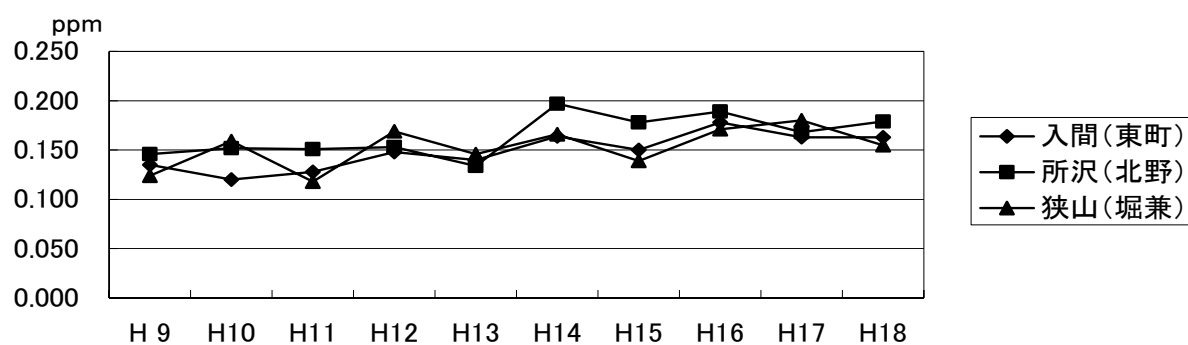
■ 光化学オキシダントの測定結果(昼間の1時間値の最高値)
