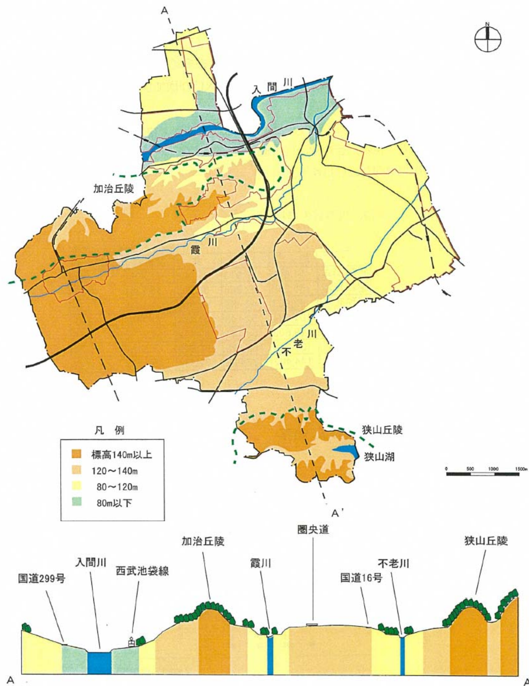
図 1-2 地形概要図及び地形概略断面図
