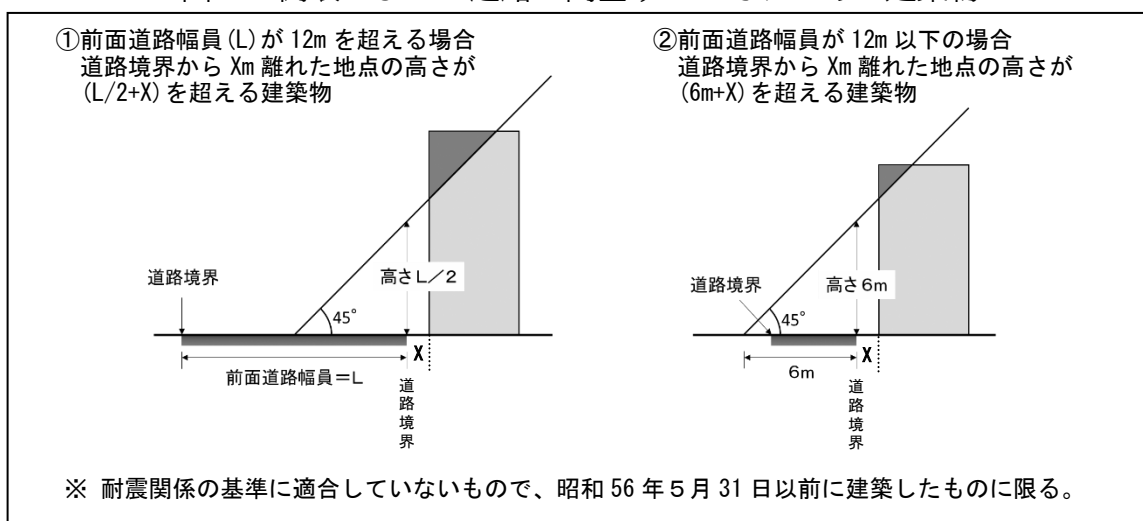
図1 倒壊によって道路を閉塞するおそれのある建築物
