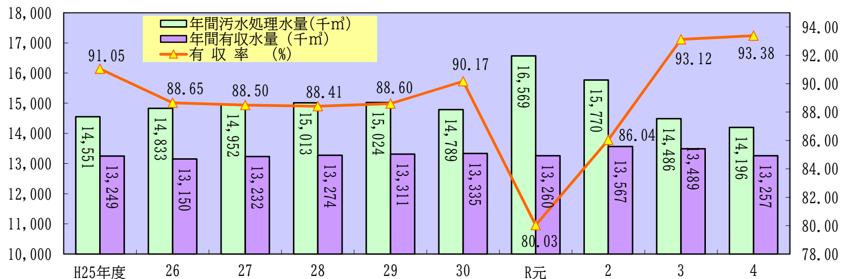
年間汚水処理水量・年間有収水量・有収率の推移
