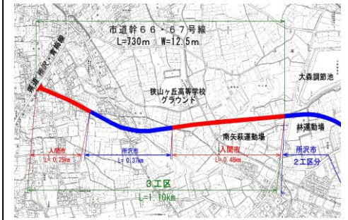
上藤沢・林・宮寺間新設道路
